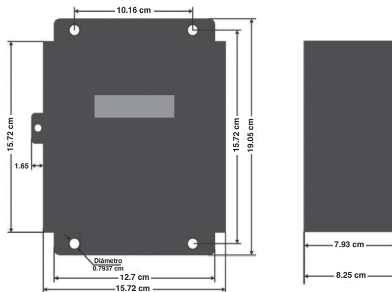
Figura 1: Dimensiones de la Caja de Acero
