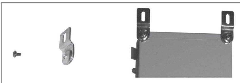
Figura 4: Montaje de la Caja
