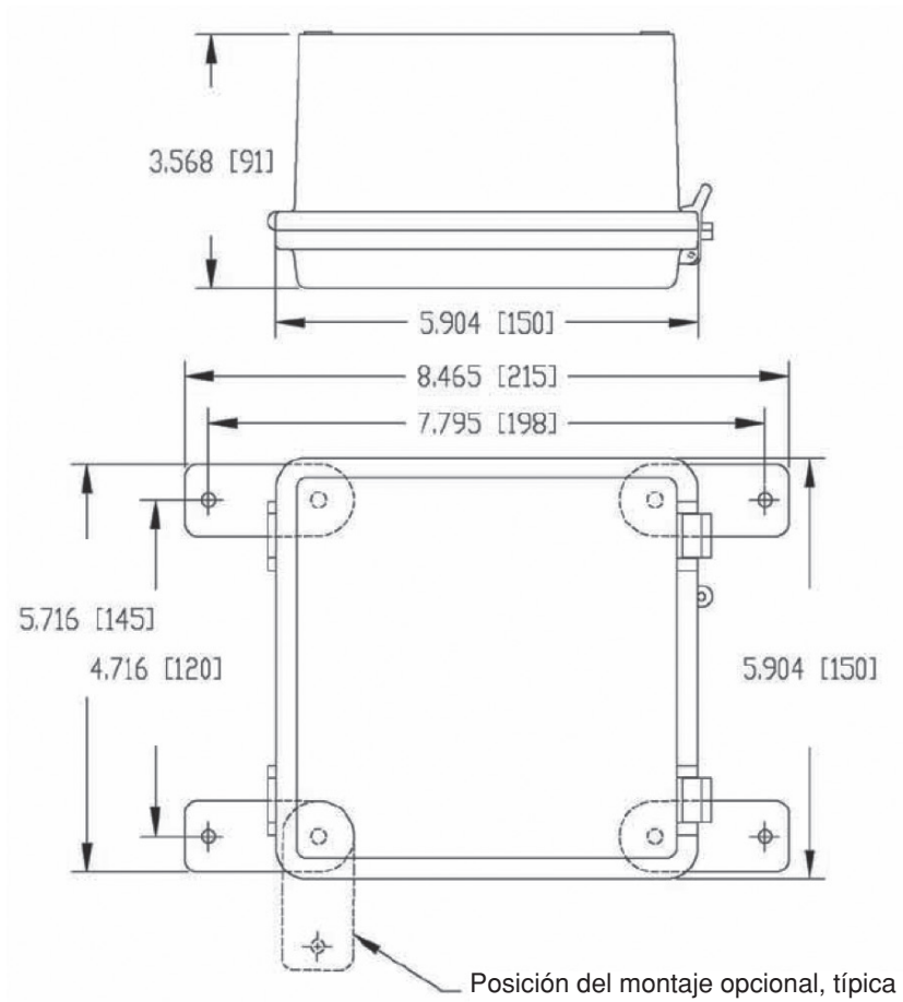
Figura 2: Dimensiones de la Caja de Plástico
