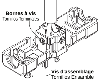
ill. 3b - Fiche lames droites Clavija de Cuchilla Recta
