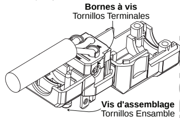
ill. 3c - Fiche équerre Clavija Angular
