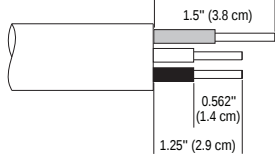
ill. 3b - Fiche lames droites Clavija de Cuchilla Recta
