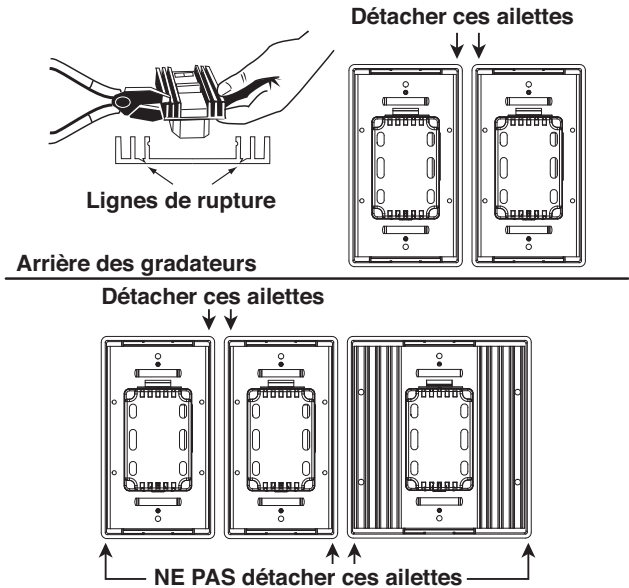
Figure 4 - Retrait des ailettes
