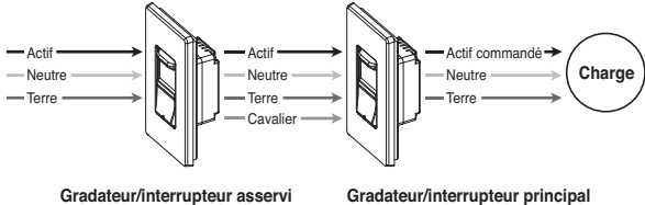
Charge après le gradateur/interrupteur asservi et le gradateur/interrupteur principal
