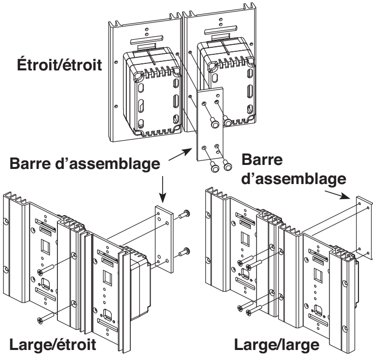
Figure 5 - Barre d'assemblage
