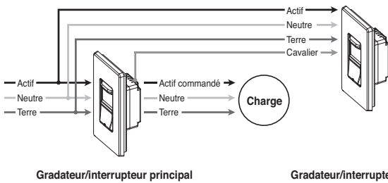
Charge entre le gradateur/interrupteur asservi et le gradateur/interrupteur principal
