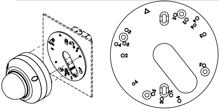
HOLE POSITION DIAGRAM 孔位圖
