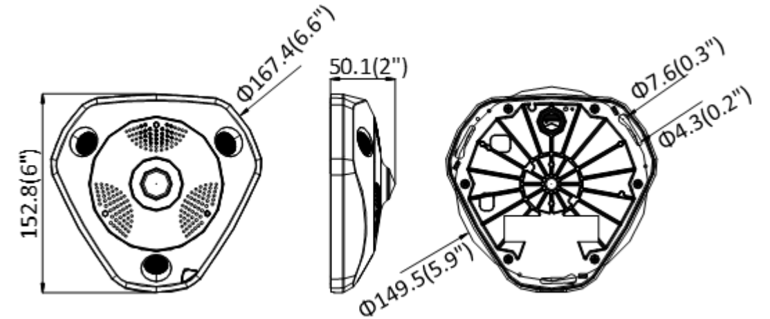
DS-2CD6365G0E-IS
