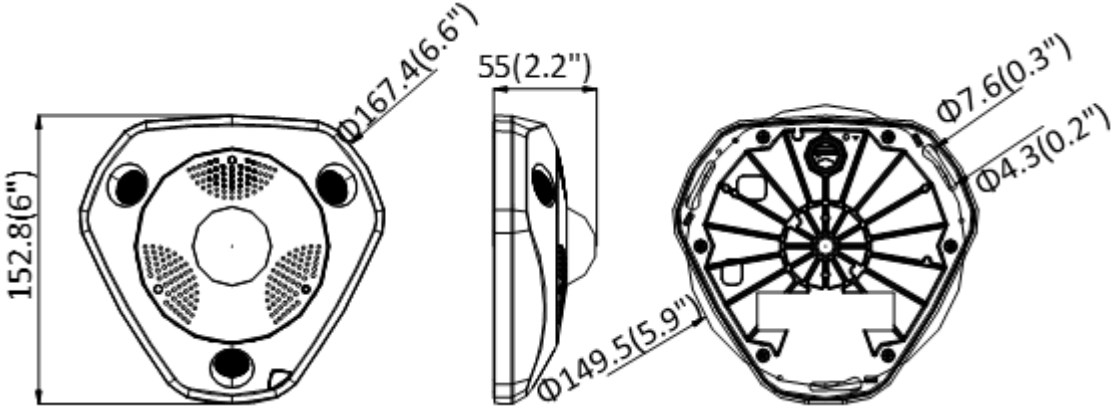
DS-2CD6365G0E-IS
