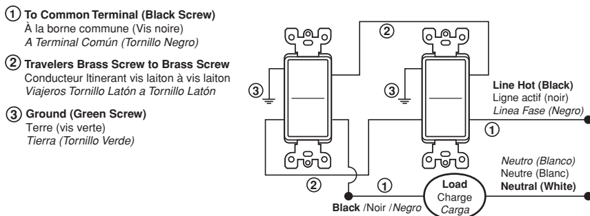
Wiring Diagram / Schéma de câblage / Diagrama de Cableado
